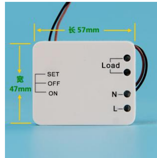
图四 产品背面结构图
