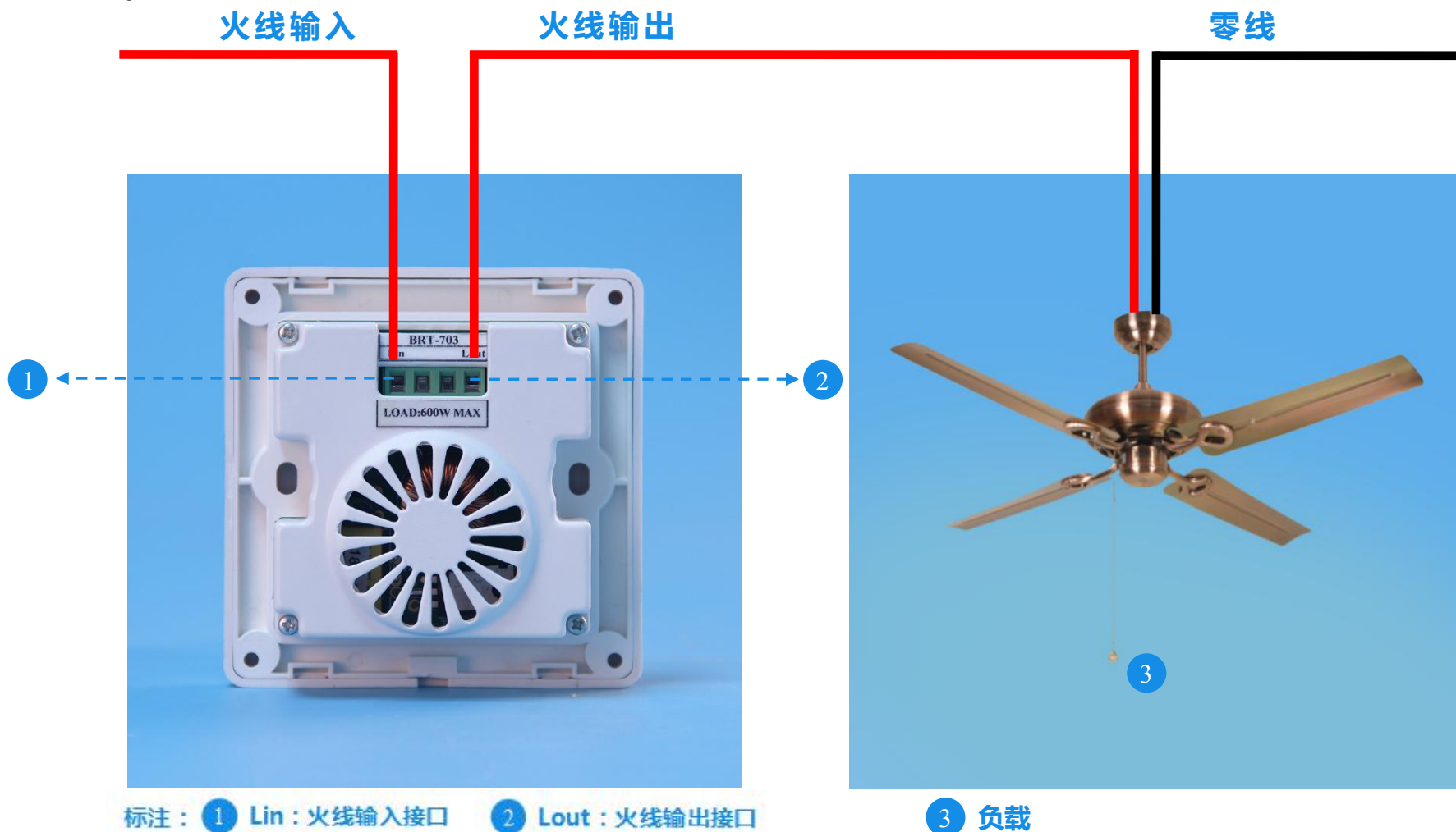
BRT-701/703 单火线接入接线示意图
